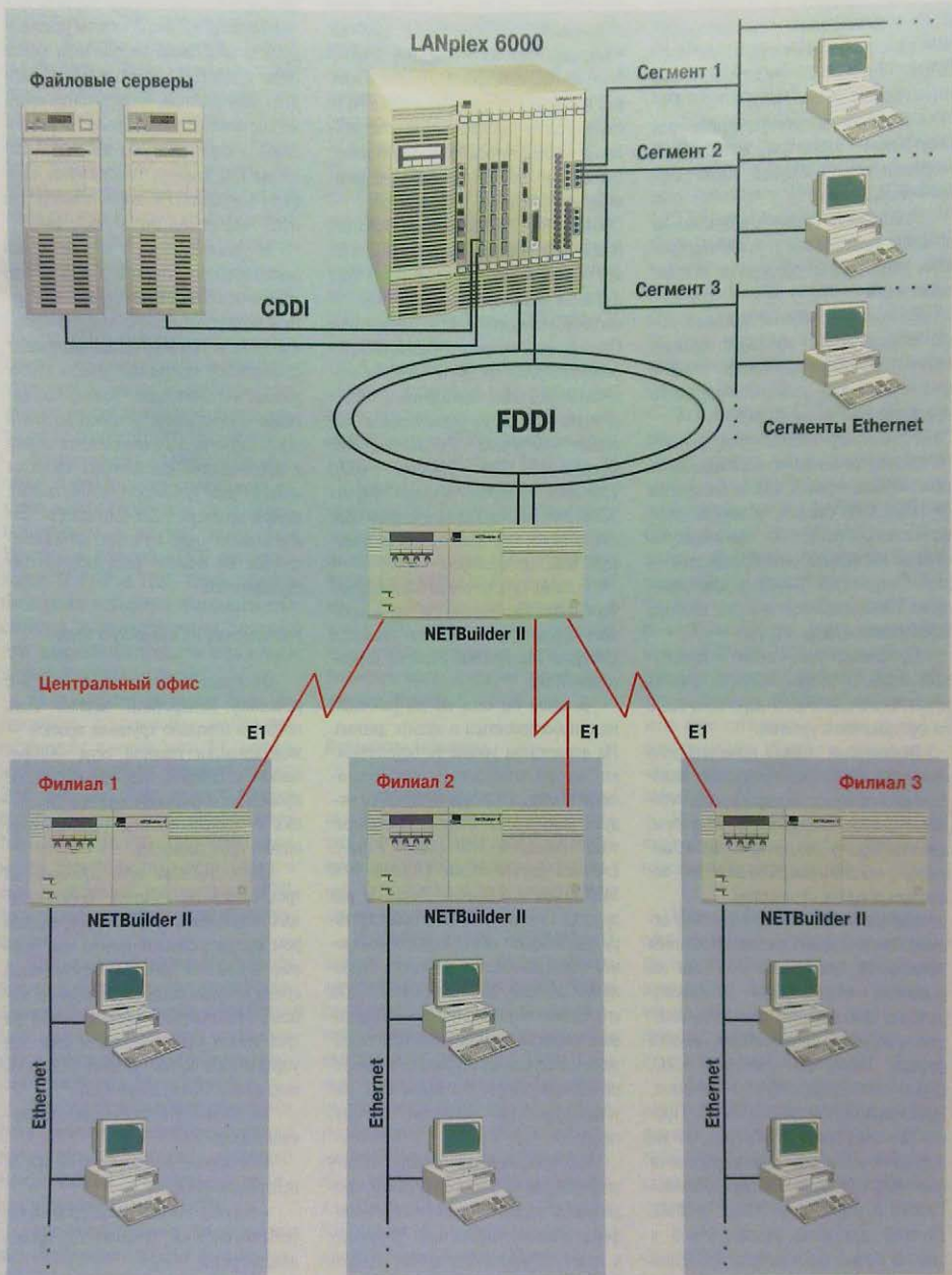
Проект сети для "Альфа-банка"
