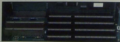
Гнездо для платы VL-Bus
